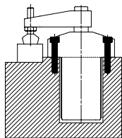
1- Montage von oben durch die Flansch mit den Innensechskantschrauben (DIN 912) 1- Mounting from above with imbus bolt through the flange
