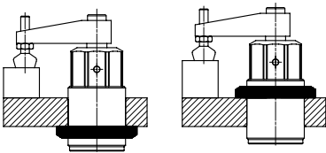
1- Montage mit Verbindungsmutter (6010-3) 1- Mounting with connection nut
